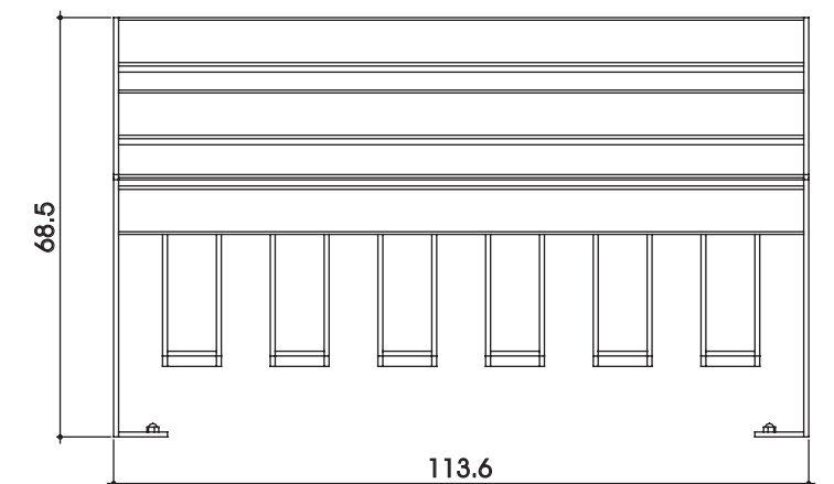
PROSPETTO
