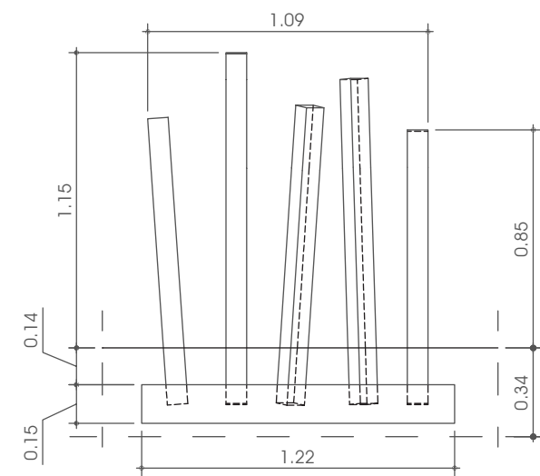
PROSPETTO
