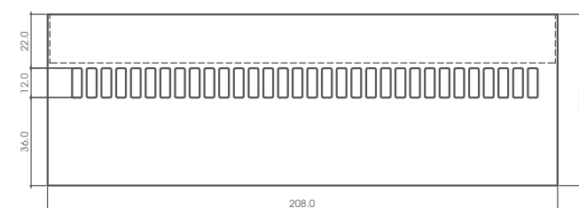
PROSPETTO
