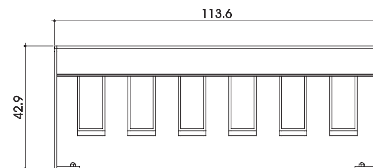
PROSPETTO
