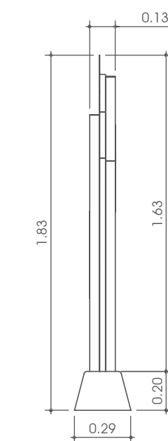
FIANCO
