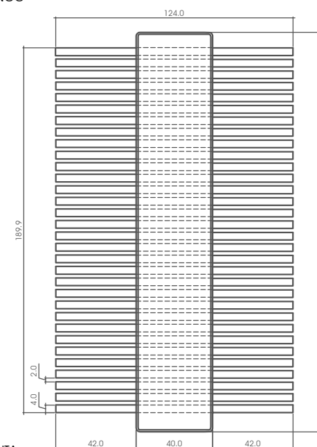
PIANTA
